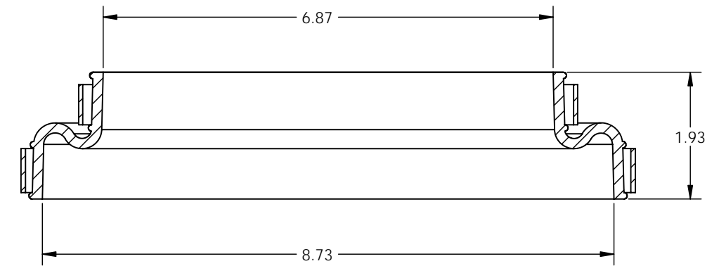
SECTION A-A
